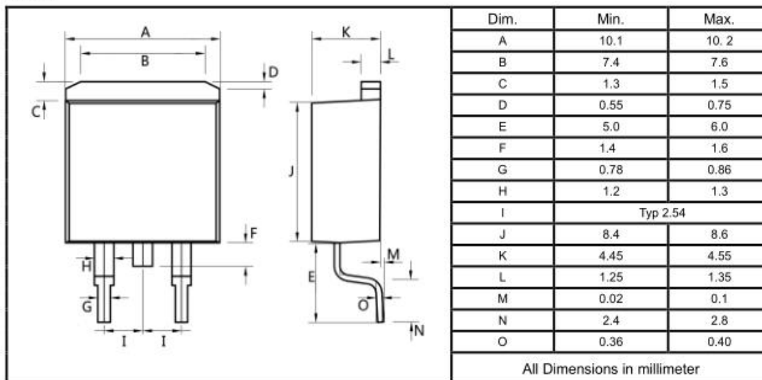
TO-263
