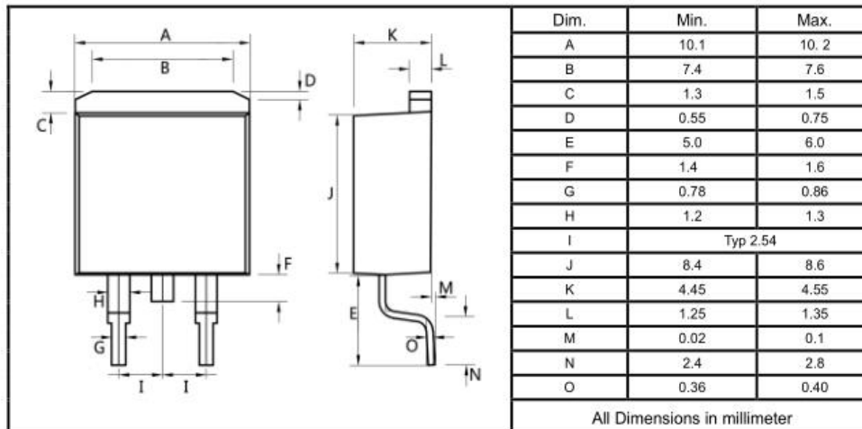
TO-263
