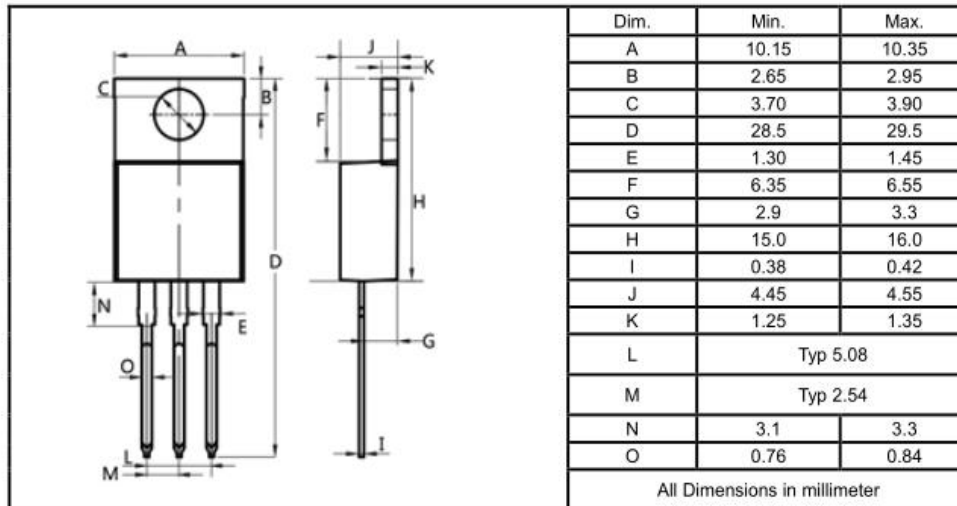
ITO-220
