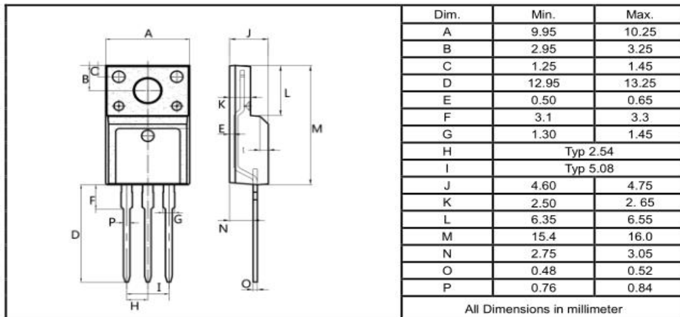
ITO-220
