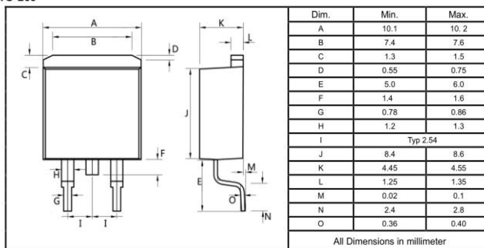
TO-263
