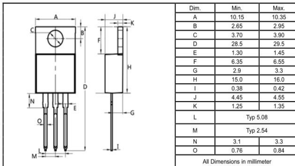
ITO-220
