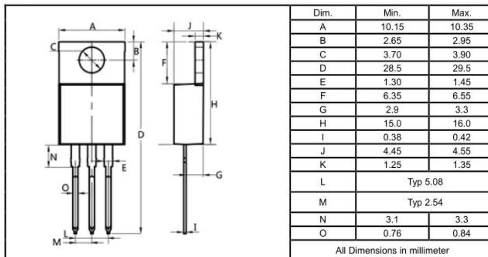
ITO-220
