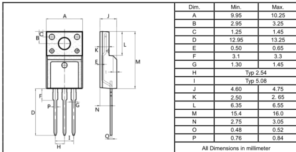
ITO-220
